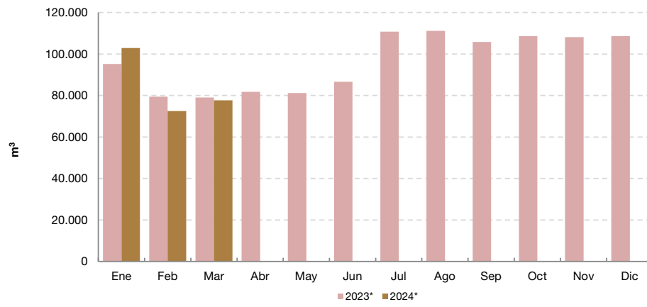
Gráfico 3.4 Producción de bioetanol, en m 3 . Enero 2023-marzo 2024
