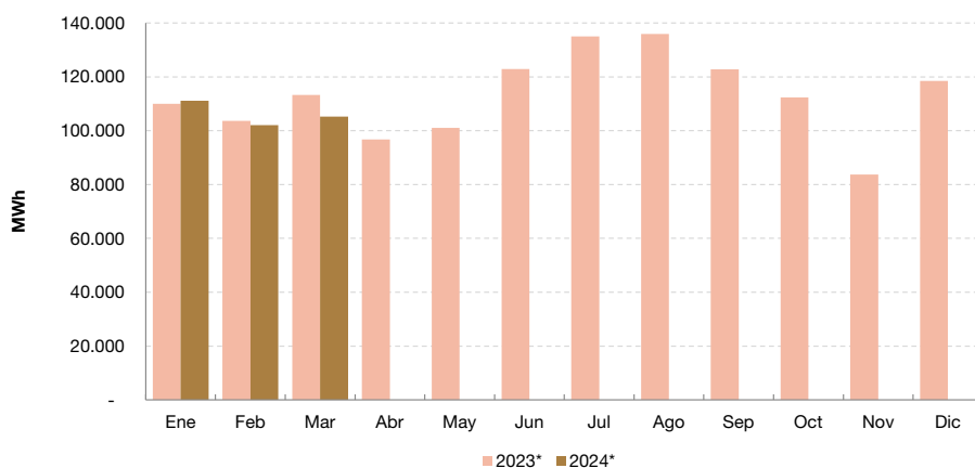
Gráfico 2.4 Energía cogenerada total en MWh. Industria manufacturera. Enero 2023-marzo 2024
