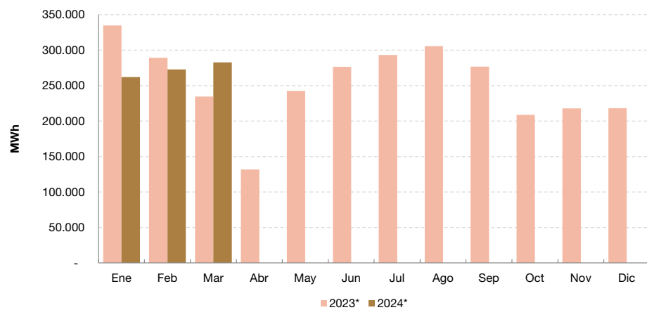
Energía autogenerada despachada al MEM en MWh. Minería e industria manufacturera. Enero 2023-marzo 2024
