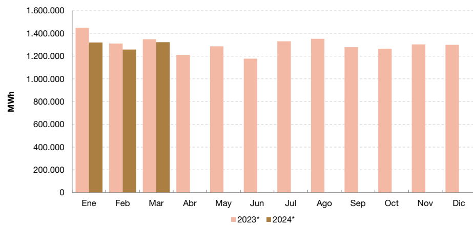
Energía autogenerada total en MWh. Minería e industria manufacturera. Enero 2023-marzo 2024
